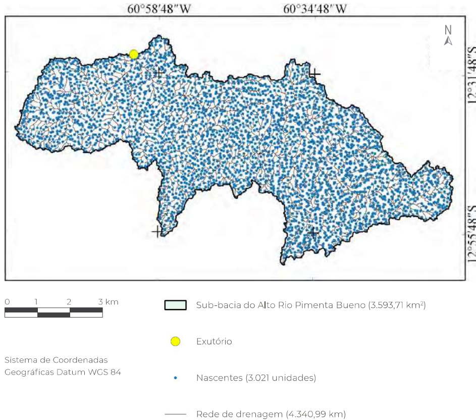
Figura 5 Distribuição espacial das nascentes na sub-bacia do Alto Rio Pimenta Bueno, Amazônia Ocidental, Brasil
